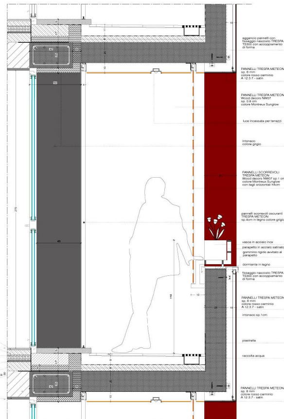
DETTAGLIO DI FACCIATA - Involucro trasparente e balcone Sezione verticale AA - scala 1:10
