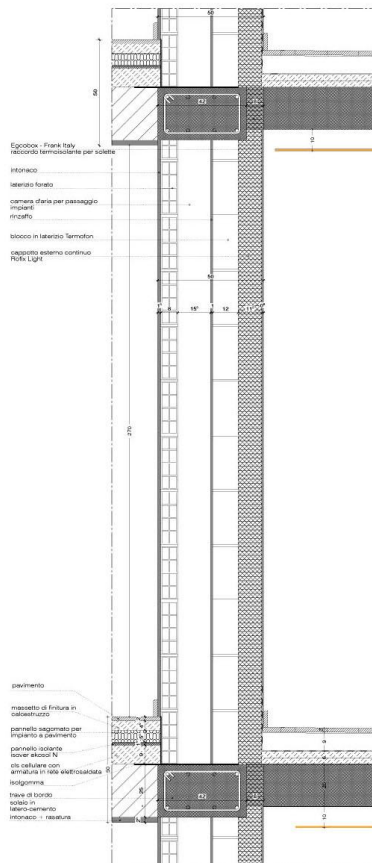
DETTAGLIO DI FACCIATA - Involucro opaco Sezione verticale BB - scala 1:10
