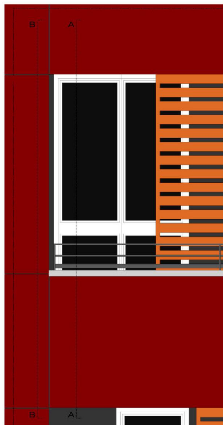
DETTAGLIO DI FACCIATA Prospetto - scala 1:10
