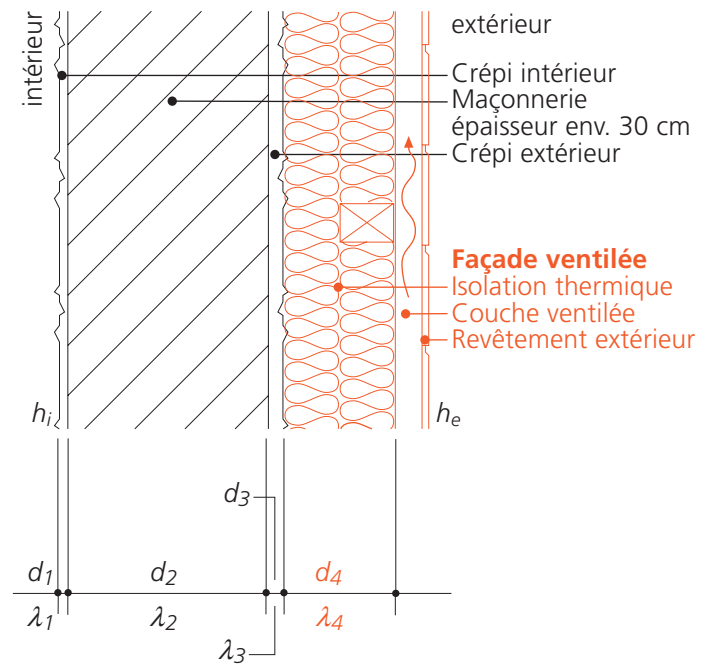
Fig. 8 Façade ventilée
